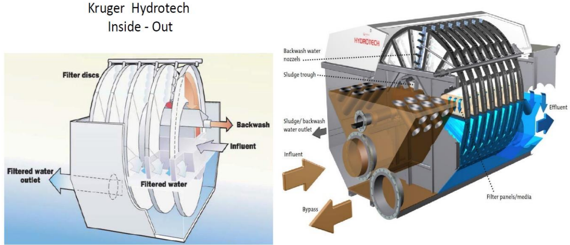
شكل 10 : عملية الترشيح خلال وحدة الترشيح In-Ou
