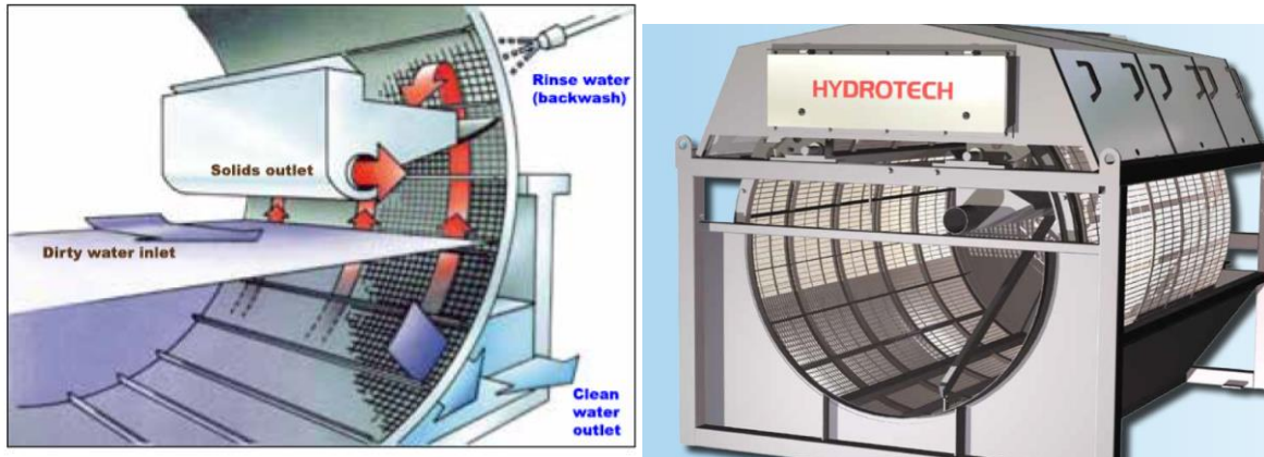
شكل 7 : مرشح أسطواني
