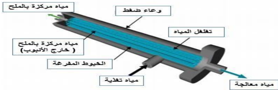
شكل 20 - الأغشية ذات الخيوط المفرغة المستخدمة في عمليات التناضح العكسي
