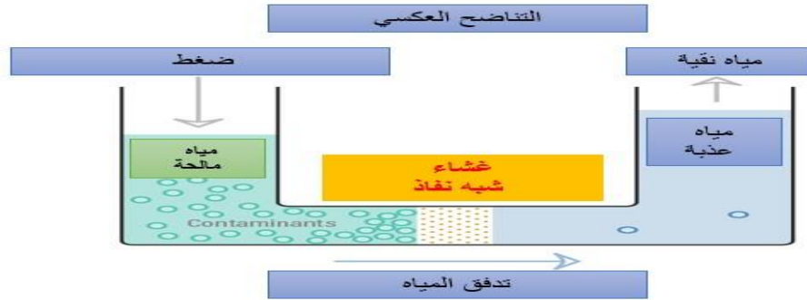
شكل 18 - شكل توضيحي يبين تنقية التناضح العكسي
